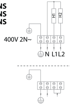
Kuva 9 Fig.9 Tekniset tiedot Technical Data
