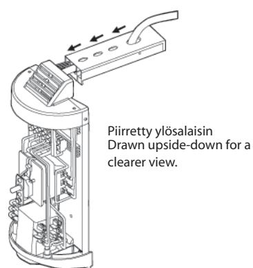
Kuva 4 Kaapelin yhdistäminen Fig. 4 Cable Connection
